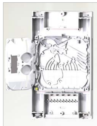
ODZS EK 330 vnitřní pohled
