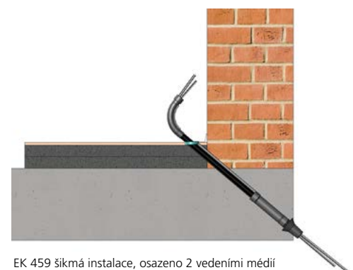
EK 459 šikmá instalace, osazeno 2 vedeními médií
